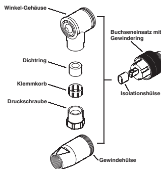
Stecker/Buchse M12
