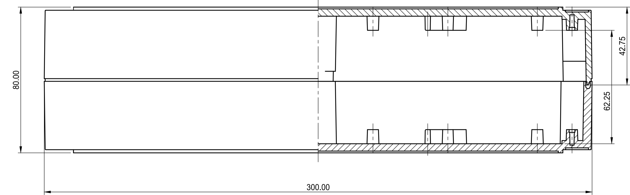
Schnitt A-A section
