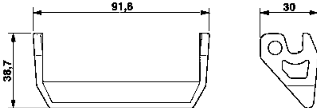
Maßzeichnung
