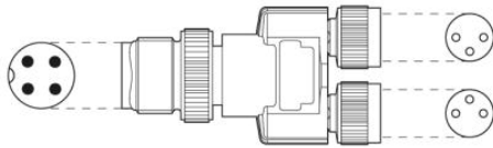
Poolschema steker M12, 4-polig, A-gepolariseerd, aanzicht stiftzijde
