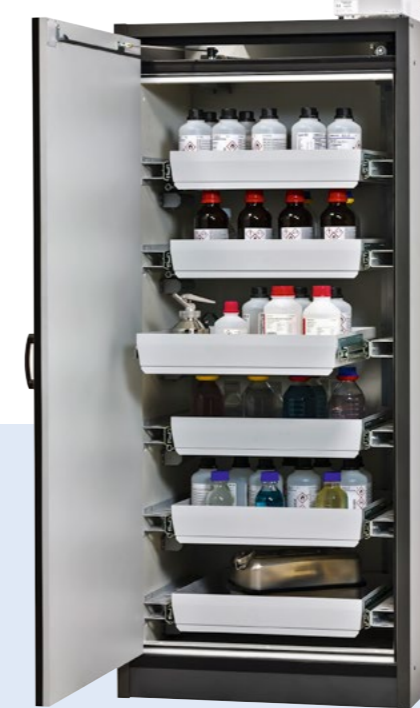
Perfekten Zugriff auf den gesamten Schrankinhalt bietet die große Flügeltür, hier am Beispiel des 864 mm breiten Basis-Line Typ 30-96.
