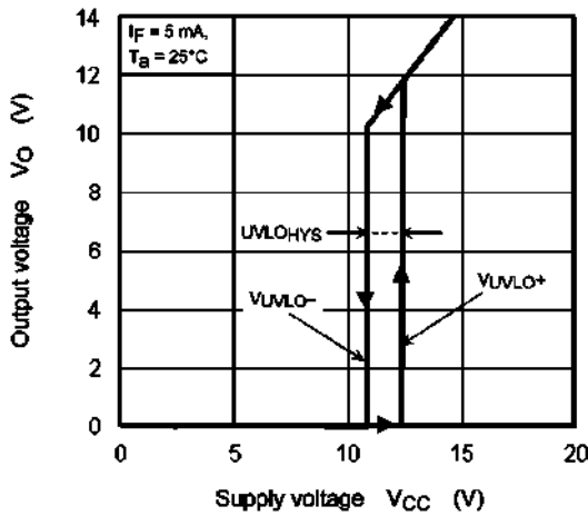
Fig. 13.2.11 V_O(V_{UMLO}) - V_{CC}
