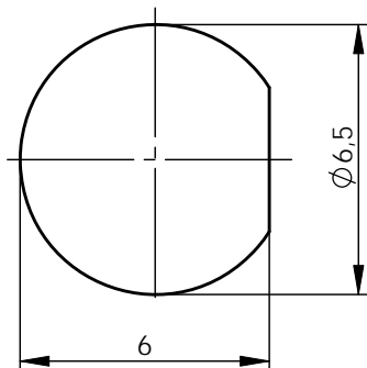
mounting dimensions / Montageausschnitt: Z 036
