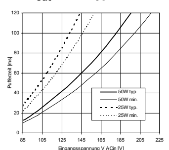
Pufferzeit bei ACin (bei V_{out} = 12\text{V} , typ. und min.)
