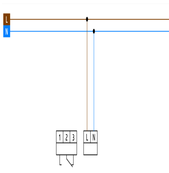
Schakelschema
