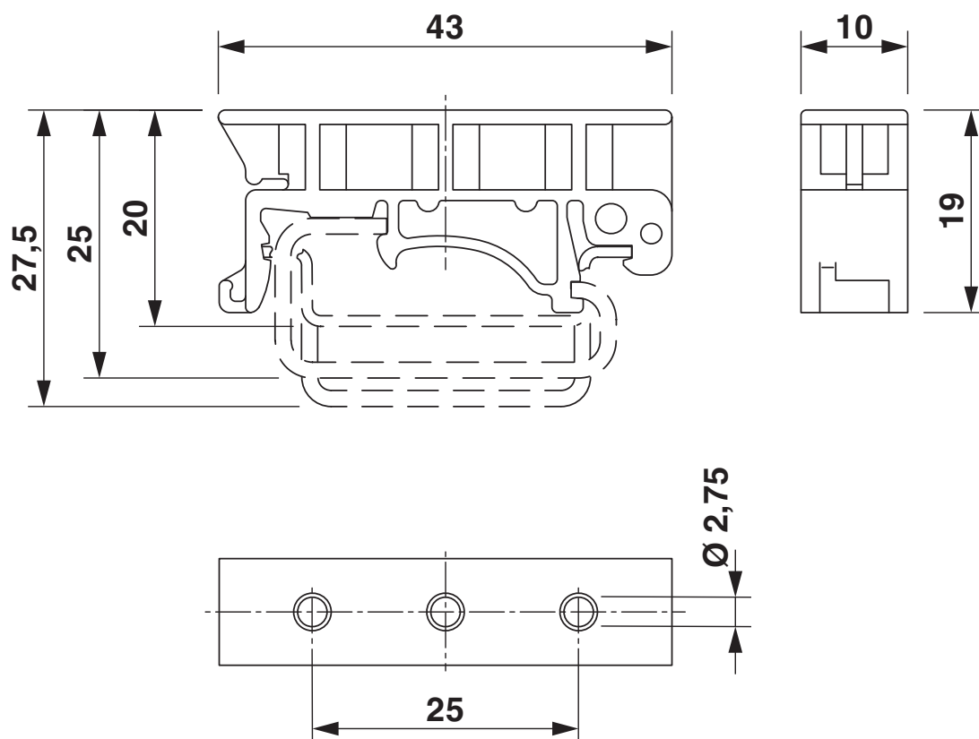
Maßzeichnung
