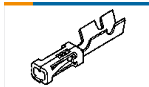
TE Teilenummer87809-1 MOD V RECP PLTD 30 AU
