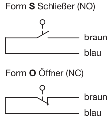
Form S Schließer O Öffner
