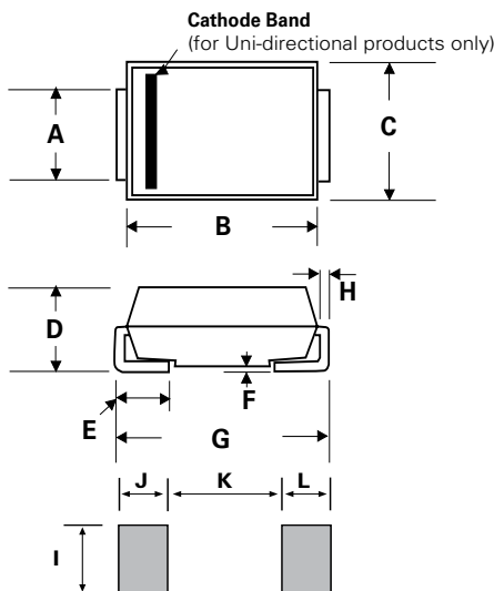
DO-214AB (SMC J-Bend)
