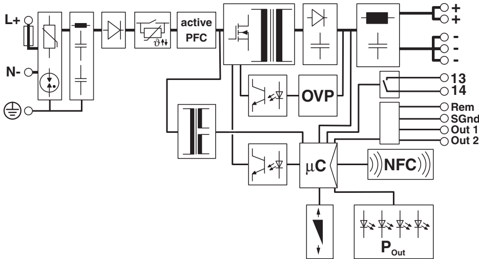
Bild 6 Blockschaltbild
