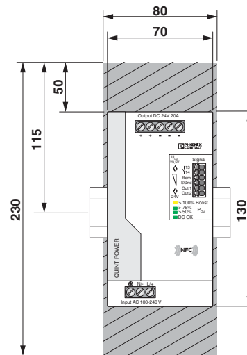
Bild 4 Geräteabmessungen und maximale Sperrflächen (Maße in mm)
