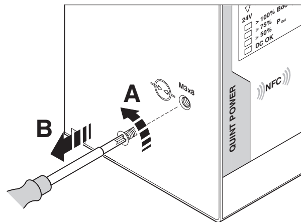
Bild 2 Gasableiter dekontaktieren
