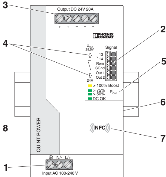
Bild 3 Bedien- und Anzeigeelemente
