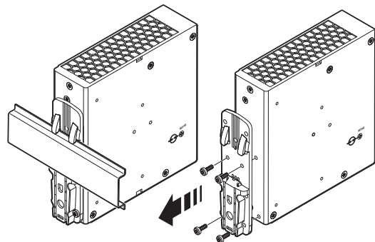
Bild 9 Universal-Tragschienenadapter demontieren
