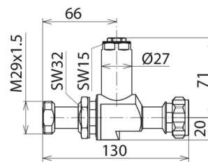
Maßbild DGA LG 7 16 MFA
