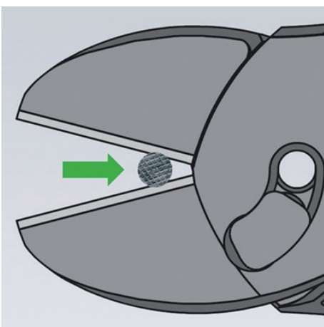
Kerf met de KNIPEX TwinForce de draad eerst in tot de noodzakelijke handkracht sterk toeneemt. Nu opent u de tang en schuift u daarbij de draad in de inkeping verder naar het scharnier toe.
