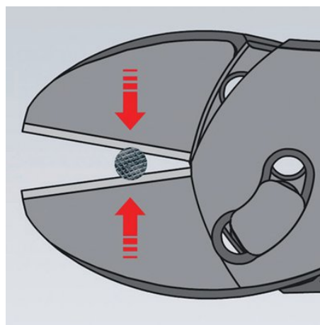
Draden legt men altijd zo kort mogelijk bij het scharnier. Bij kracht-zijsnijtangen met een hoge transmissie is de opening kort bij het scharnierpunt meestal kleiner dan de draad dik is en de draden kunnen bij het knippen naar voren glijden.
