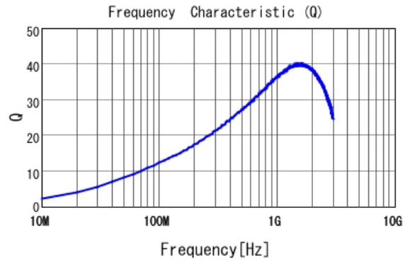
■ LQP03HQ18NH02 Q
