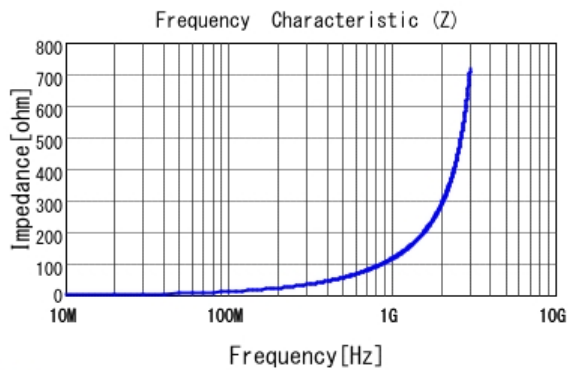
■ LQP03HQ18NH02 |Z|
