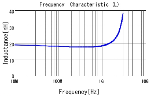
■ LQP03HQ18NH02 L
