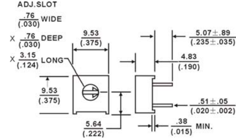
TSR-3386F
