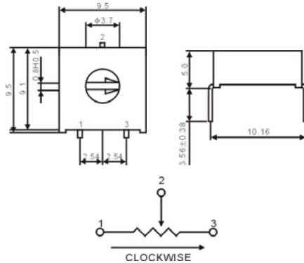
TSR-3386G
