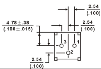
TSR-3386R
