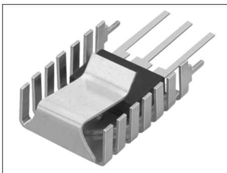
FK 245 MI 247 V 19,7 K/W mit Lötflanke für vertikalen Einbau
