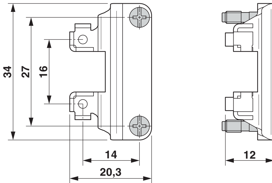
Maßzeichnung
