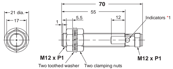
E2E-X□L18-M1
