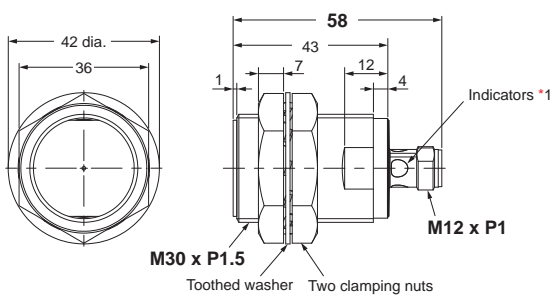
E2E-X□30-M1
