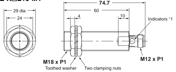
E2E-X□L30-M1
