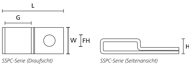
SSPC-Serie (Draufsicht)
