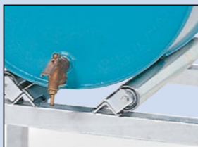
Rollenauflage für die liegende Fasslagerung, Bestell-Nr. 114-542-10
