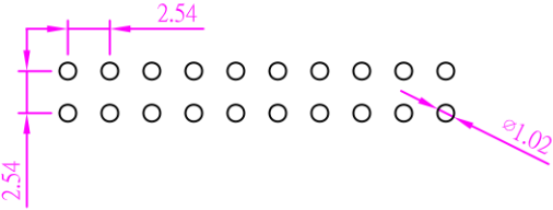
Leiterplattenbohrbild
