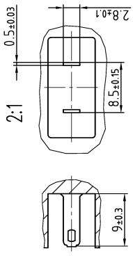
Maße für Steckeranschluss
