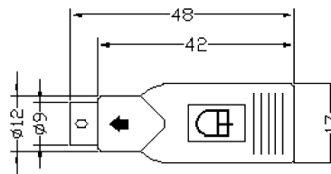
MINI DIN6 MALE INSULATOR: GREEN
