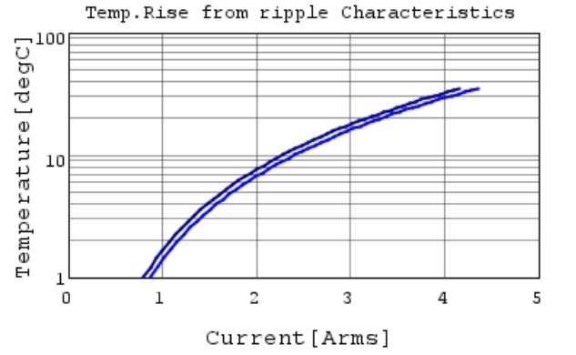
GRM188R6YA475KE15 Temp.rise — 500kHz
