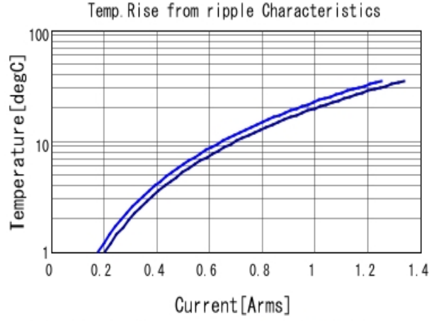
GCM155L8EH104KE07 Temp. rise ■ 800kHz ■ 1MHz
