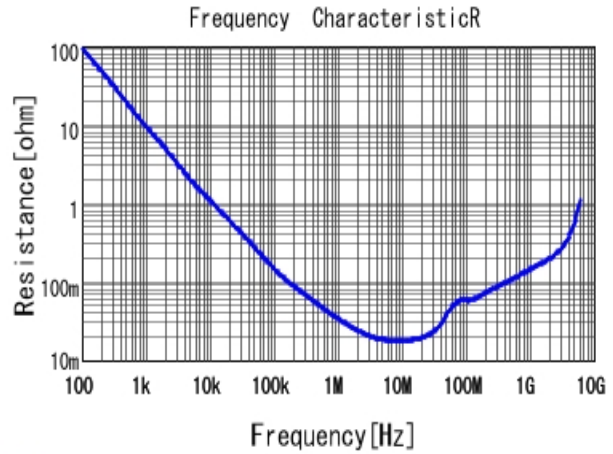
GCM155L8EH104KE07 R DCOV, 25degC
