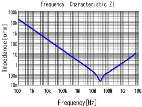
GCM155L8EH104KE07 |Z| DCOV, 25degC
