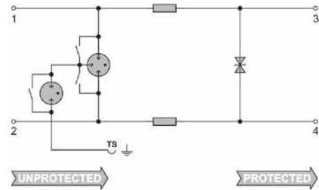
Prinzipschaltbild
