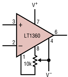
1360 A101
