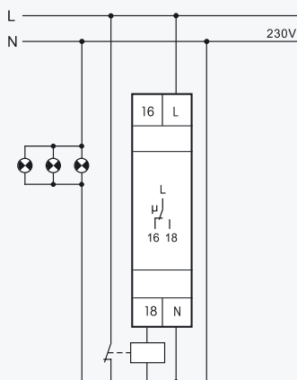
Ansteuerung der Notleuchten über Schaltschütz I > 16 A
