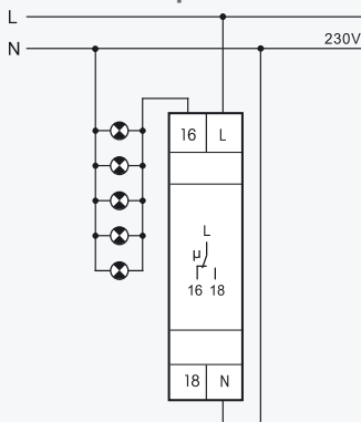
Direkte Ansteuerung der Notleuchten I \leq 16 A
