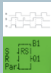
Selbsthalter-relais
