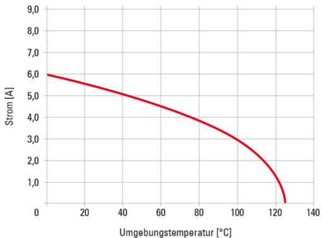
Stromtragfähigkeit Signalkontakte
