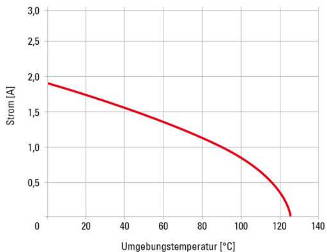
Stromtragfähigkeit Signalkontakte
