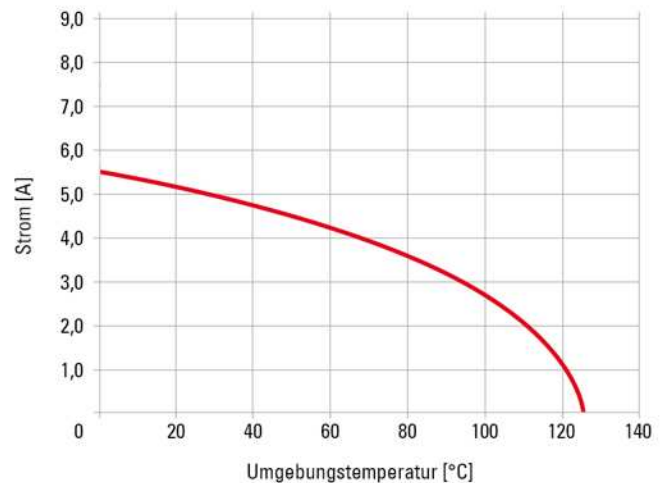
Stromtragfähigkeit Signalkontakte
