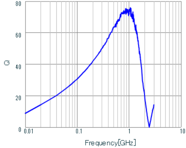
LQW18AN75NG00 Q.
