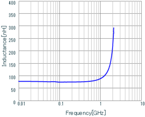
LQW18AN75NG00 L.
