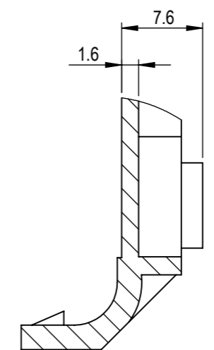
DETAIL Y SCALE 2 : 1
