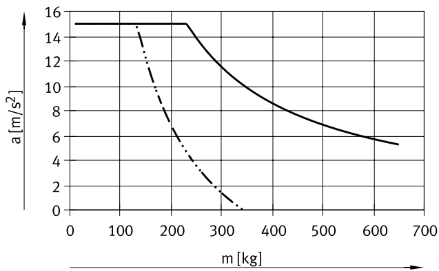
Baugröße 120
