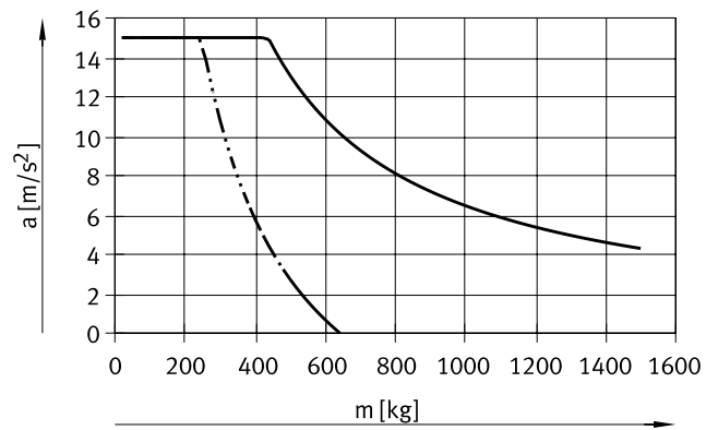
Baugröße 150
