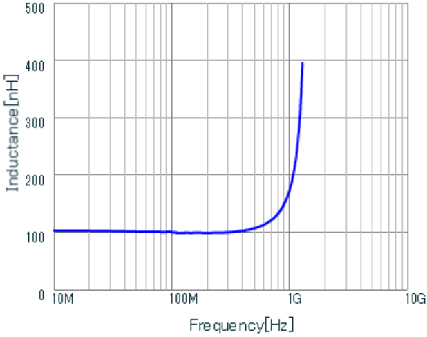
LQP03HQR10H02 L.
