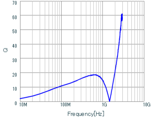
LQP03HQR10H02 Q.
