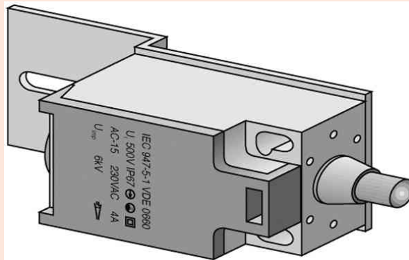
Türkontaktschalter
