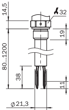
Maßzeichnung Gehäuse
