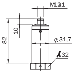
Maßzeichnung Gehäuse
