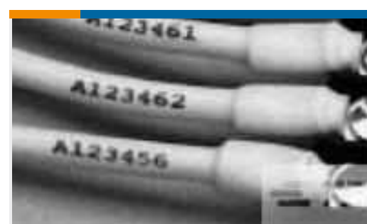
TE Teilnr.:5054324002 RNF-100-1-1/2-3-SP
