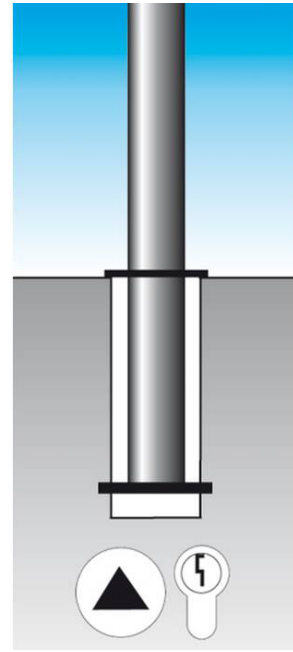
Technische Ansicht: Herausnehmbar mit DK oder PZ (inkl. Bodenhülse) Art. - Nr. 13375 o. 13376
