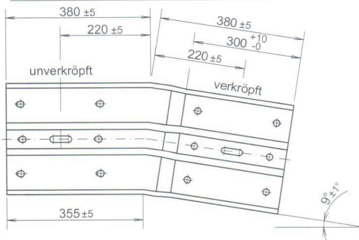
Teil Nr.13.11 Absenkwinkel B links
