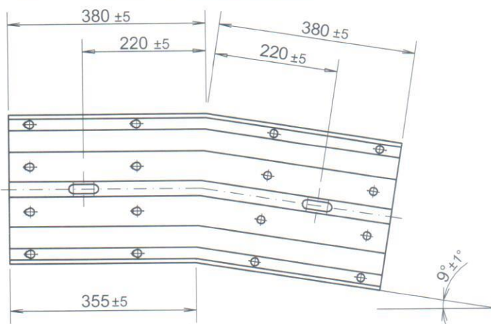
Teil Nr.13.01 Absenkwinkel A links
