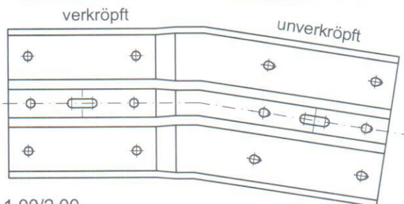
Teil Nr.13.11 Absenkwinkel B links
