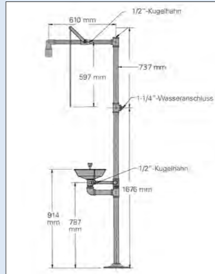
Diese Skizze gilt für die Notduschen der Typen G 1931, G 1902-P, G 1902, G 1991
