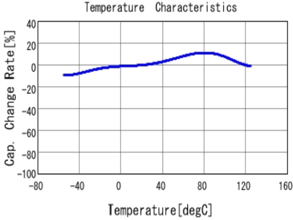
■ GRT155R71A474KE01 C-Temp. capchange, DCO. 0V, ACO. 5V rm
