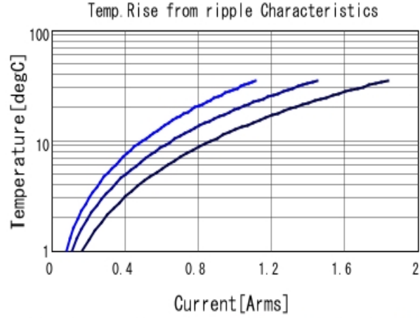
GRT155R71A474KE01 Temp. rise ■ 200kHz ■ 500kHz ■ 1MHz
