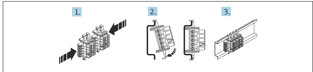
2 Montage Tragschienen-Busverbinder 12,5 mm (0,5 in)
