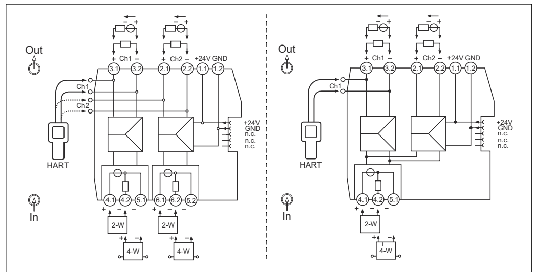
8 Klemmenbelegung: 1- und 2-Kanal Version (links), Signaldoppler (rechts)
