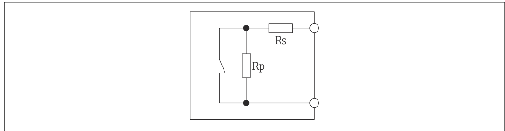
22 Widerstandsbesaltung zur Leitungsüberwachung (Kurzschluss und Unterbrechung)
