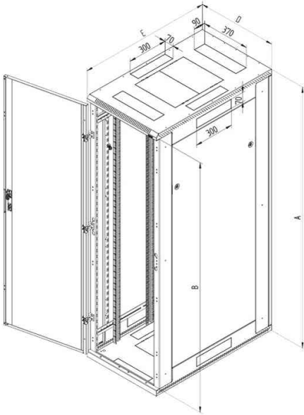
Symbolzeichnung: 19" Netzwerkschrank RJA, geöffnet
