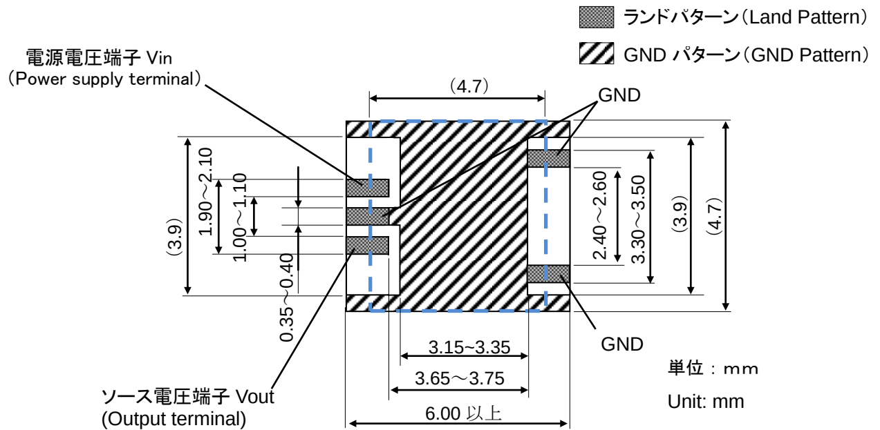
図6 標準ランドパターン
