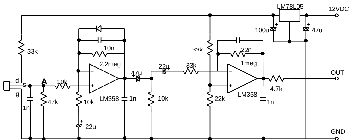
図3 標準測定回路
