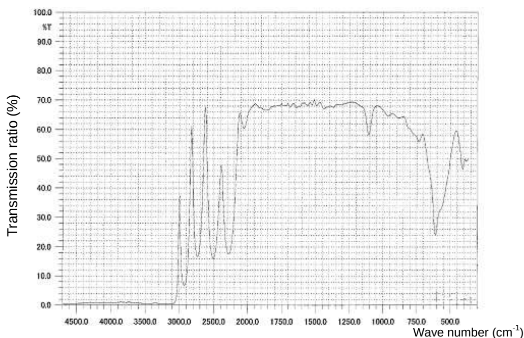
図5 赤外線透過特性例
