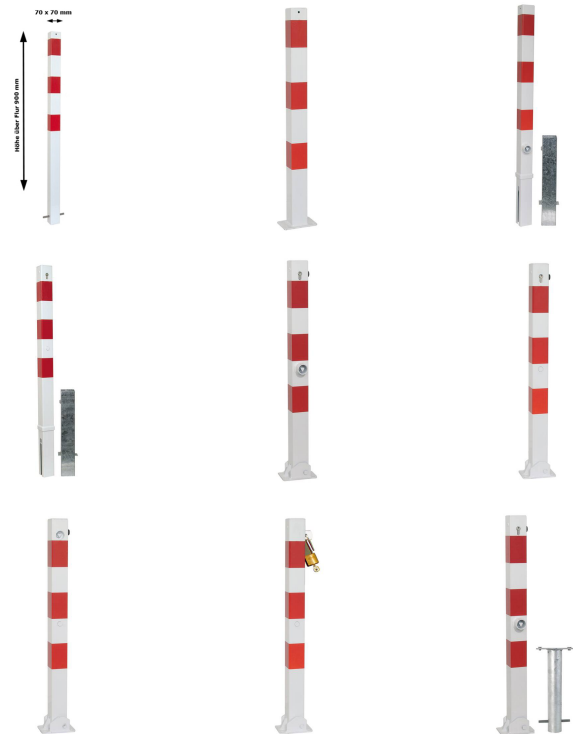
Modellbeispiele: Absperrpfosten -Bollard- 70x70 mm (weiß beschichtete und verzinkte Modelle)
