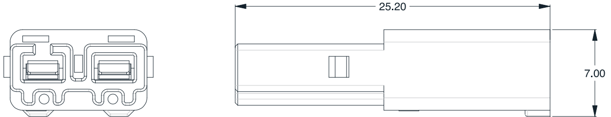
Plug (2271180-1) :
