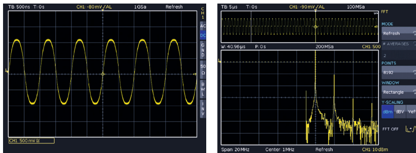
Sinussignal in der Zeitdomäne
