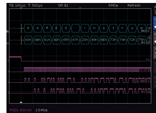
SPI Bussignal, MISO / MOSI dekodiert
