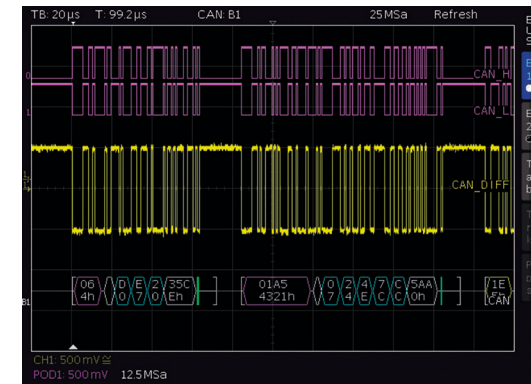
HEX dekodiertes CAN Bussignal
