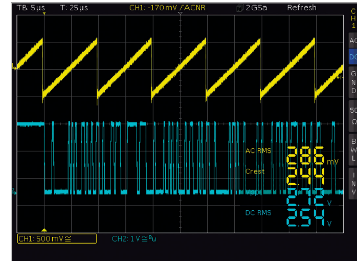
DVM auf zwei Analogkanälen mit vier Messparametern
