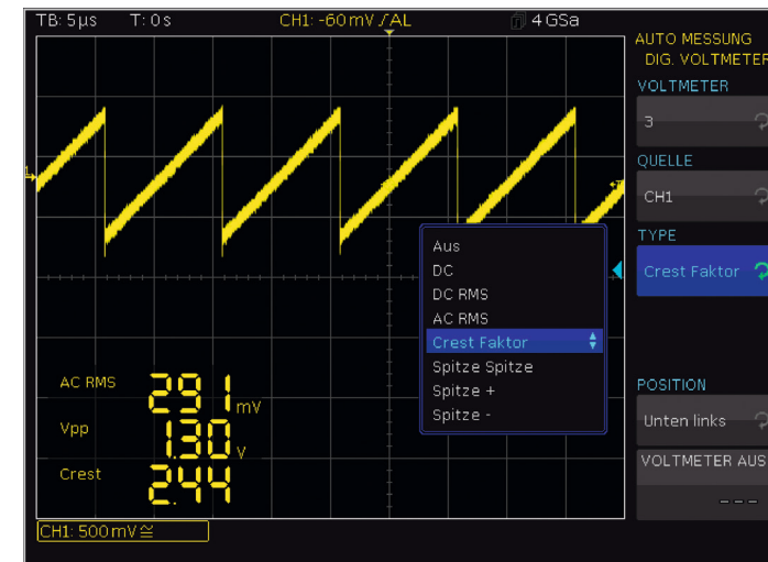
Sägezahnsignal mit DVM gemessen
