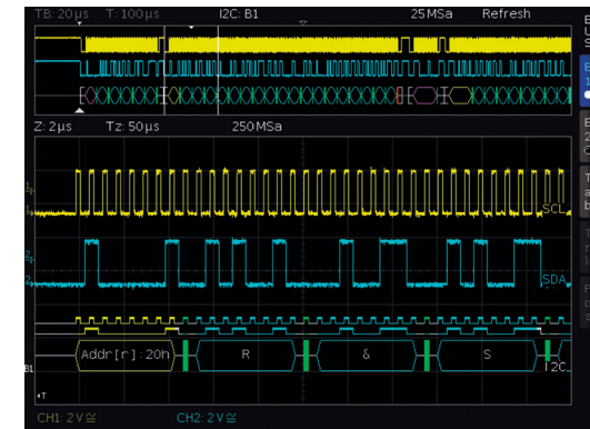
I 2 C Bussignal in Zoomansicht
